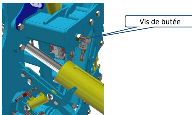
Figure 30 Butées des bras latéraux
