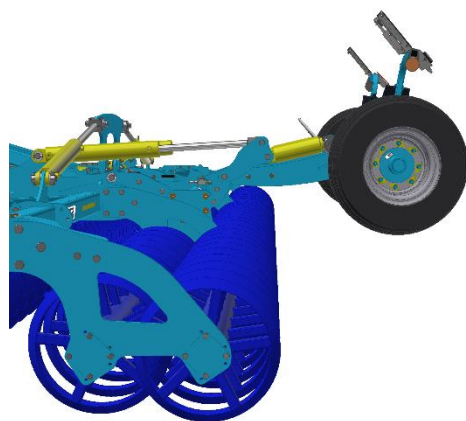
Figure 22 Position de l'essieu lors du travail
