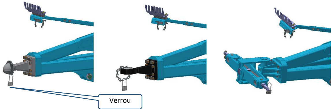
Figure 6 Dispositif contre une utilisation non autorisée
