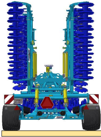
Figure 11 Position de la machine pour le dépliage
