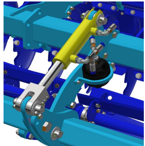
Figure 17 Tige de piston de l'outil avant
